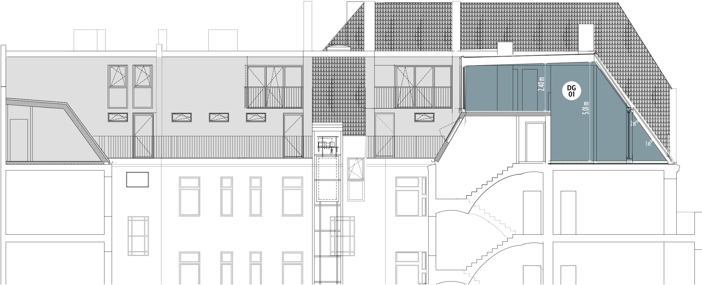
Schnitt Seitenflügel
